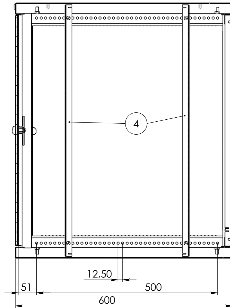
СЕЧЕНИЕ С-С
