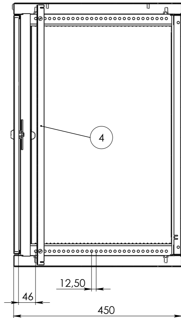
СЕЧЕНИЕ С-С
