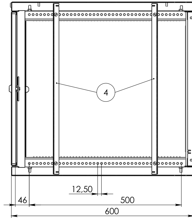
СЕЧЕНИЕ С-С
