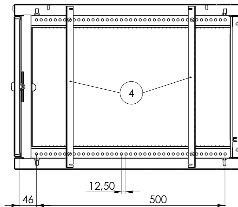
СЕЧЕНИЕ С-С
