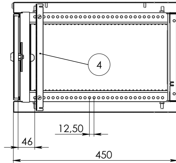
СЕЧЕНИЕ С-С
